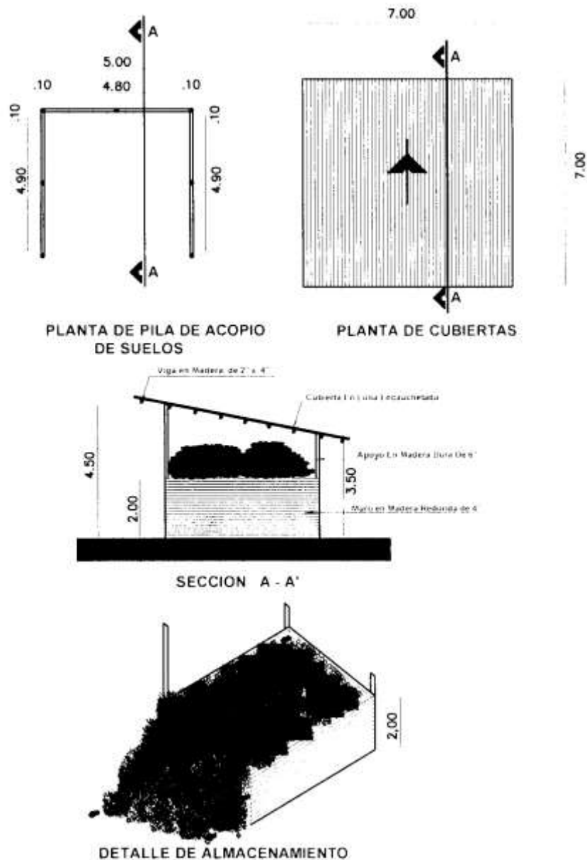
Figura 11. Acopio de suelo (capacidad 46m 3 )
